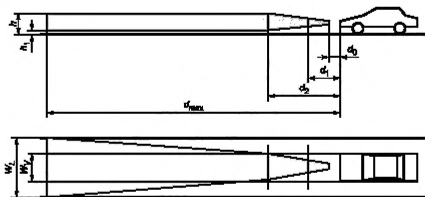
Рисунок 3 — Зона обнаружения
