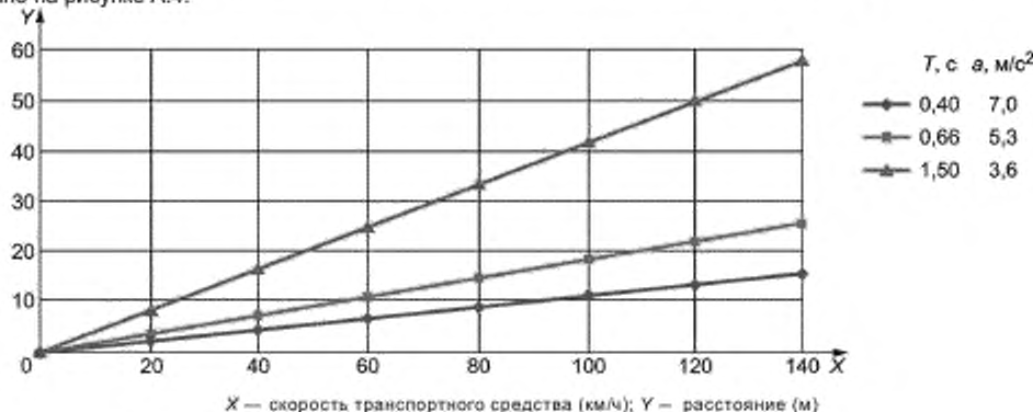
Рисунок А.4 — Отношение между скоростью транспортного средства и расстоянием, на котором выдается предупреждение о движущемся вперед с постоянной скоростью транспортном средстве
