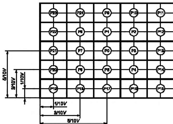
Рисунок 8 — Стандартные позиции измерений
