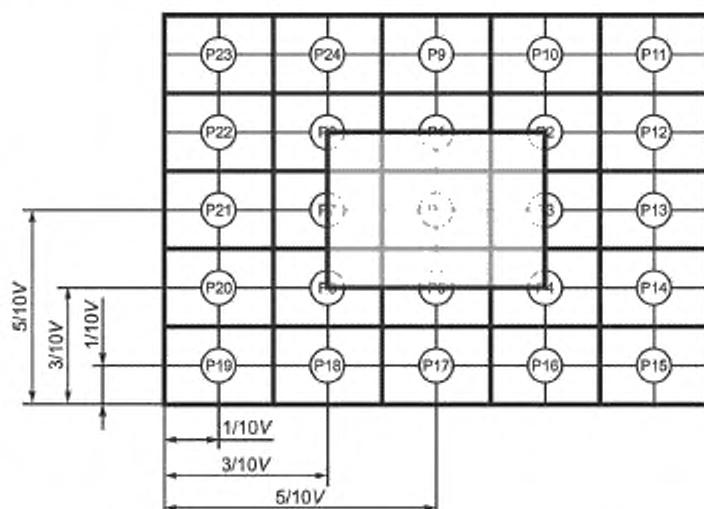
Рисунок 9 — Прямоугольное окно при измерении перекрестной помехи
