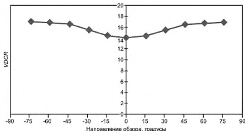
Рисунок 14 — Пример зависимости контрастности от направления обзора
