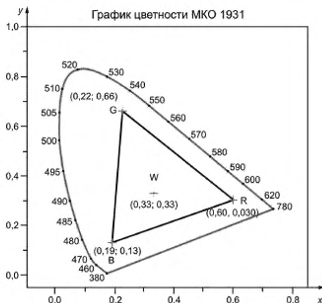
Рисунок 10 — Пример цветовой гаммы дисплея
