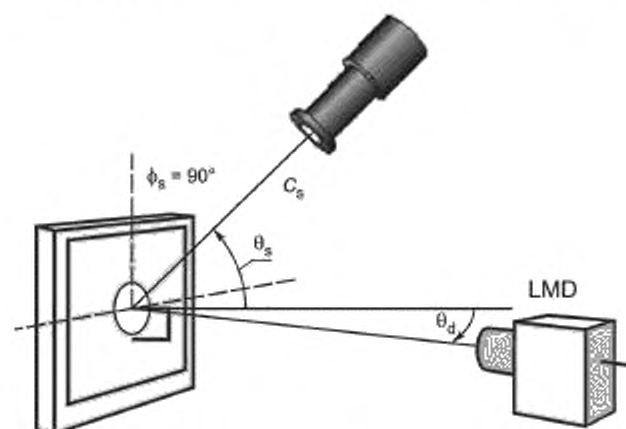
Рисунок 13 — Конфигурация освещения при измерении характеристик направления обзора спектрального отражающего дисплея
