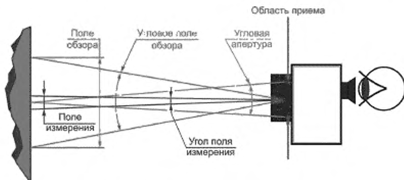
Рисунок 7 — Схема измерительной установки
