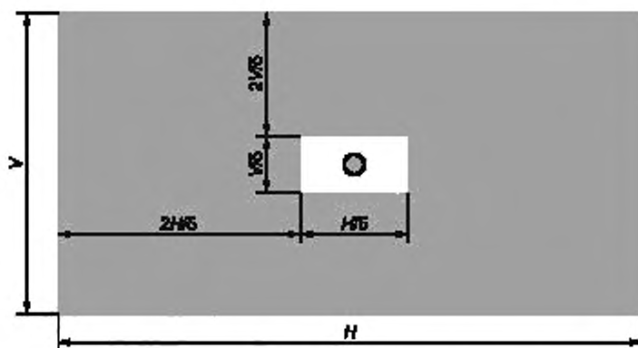
Рисунок 15 — Таблица дисплея, используемая для снятия характеристик двоения
