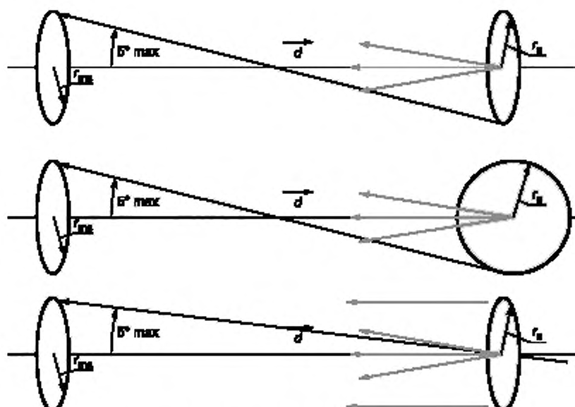
Рисунок 2 — Примеры направленного освещения
