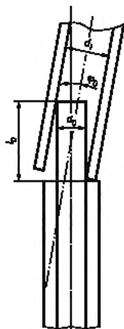
а) Угловое искажение во втулочном соединении
