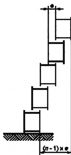
с) Смещения, приводящие к поперечным отклонениям
