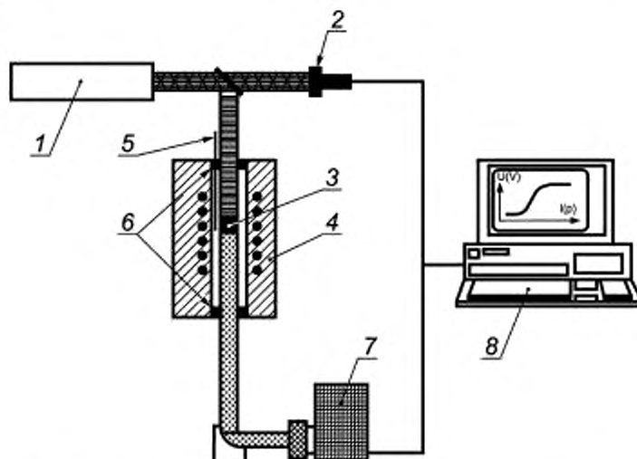
1 — импульсный излучатель; 2 — детектор импульсов; 3 — образец; 4 — печь или климатическая камера; 5 — прибор для измерения температуры; 6 — окна; 7 — детектор переходных параметров (удаленный датчик измерения температуры); 8 — устройство управления, сбора данных и анализа
