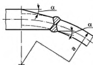
с) Соединение более тонкого днища с обечайкой
