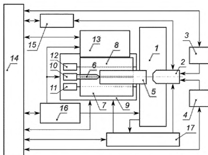
Рисунок 1 — Схема технологической установки для получения порошка методом плазменного распыления быстровращающейся заготовки
