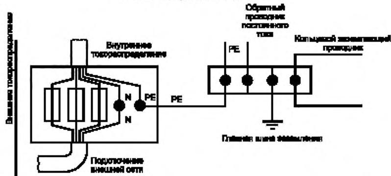
Рисунок В.2 — Принципы перехода от наружной распределительной сети к внутренней сети здания
