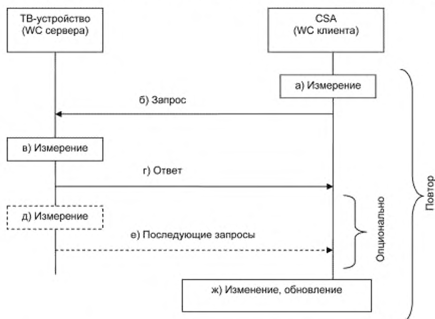
Рисунок 8 — Процедура синхронизации системных часов через интерфейс WC
