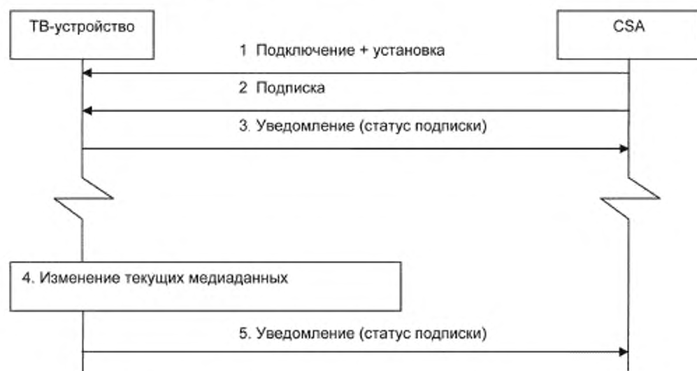
Рисунок 11 — Видоизмененная процедура получения переключающих событий
