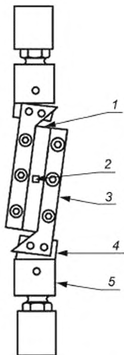
1 — образец; 2 — тензорезистор; 3 — зажимные планки; 4 — выравнивающая плитка; 5 — скоба
