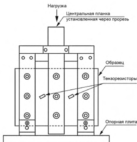
Рисунок 3 — Метод В. Эскиз приспособления
