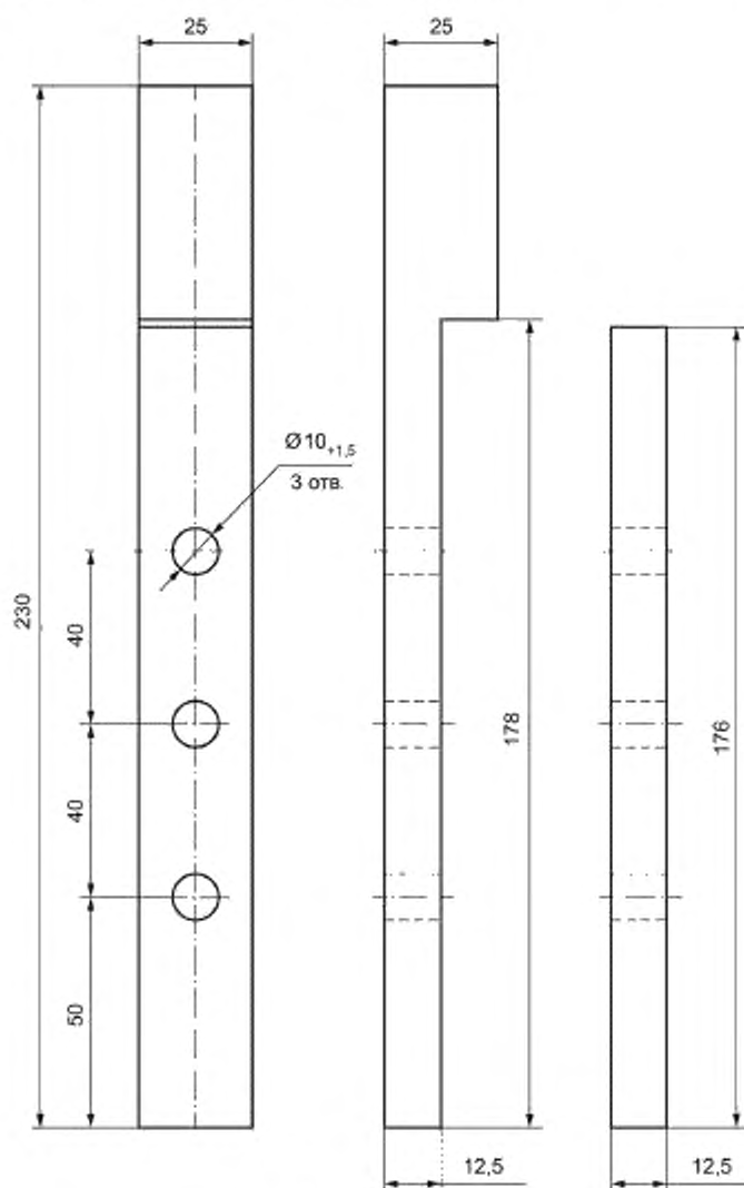
Рисунок ДБ.1 — Эскиз центральной пары планок
