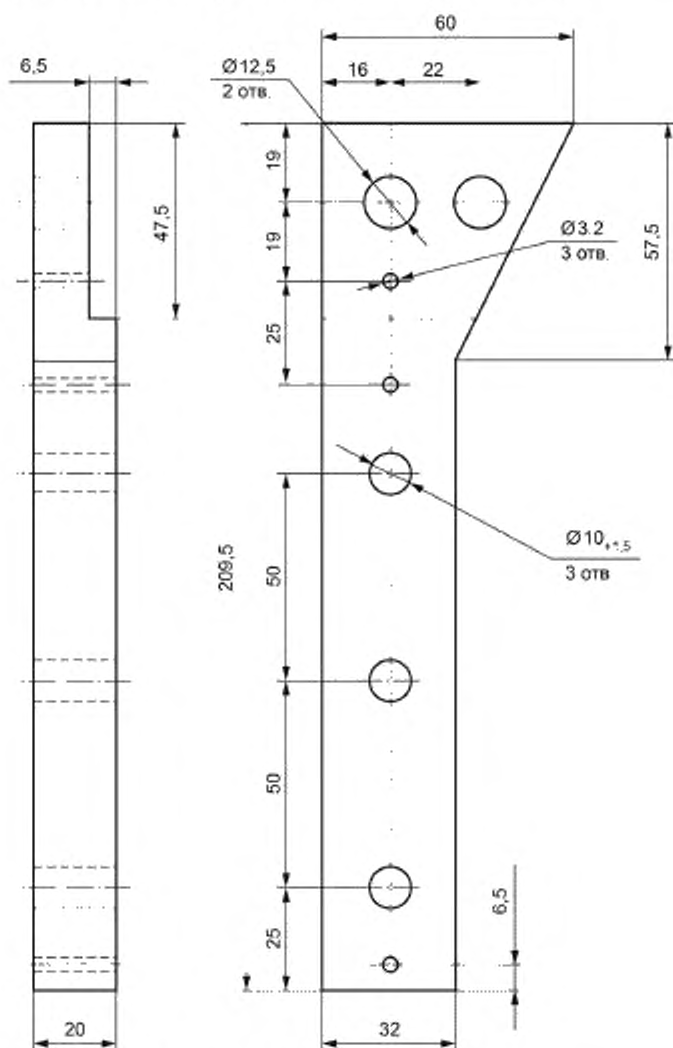
Рисунок ДА.1 — Эскиз зажимных планок
