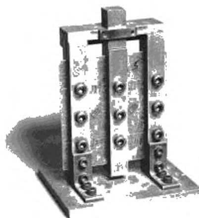
Рисунок 4 — Метод В. Фотография приспособления
