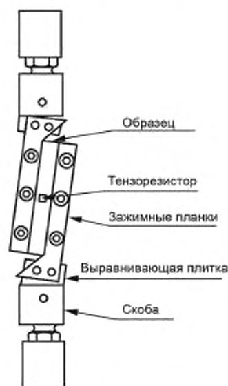
Рисунок 1 — Метод А. Приспособление для сдвига
