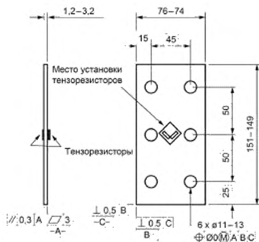
Рисунок 6 — Метод А. Образец, размеры в мм
