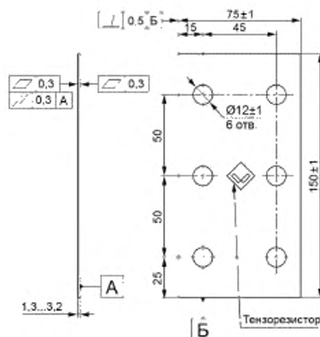
Рисунок 5 — Эскиз образца, испытываемого по методу А
