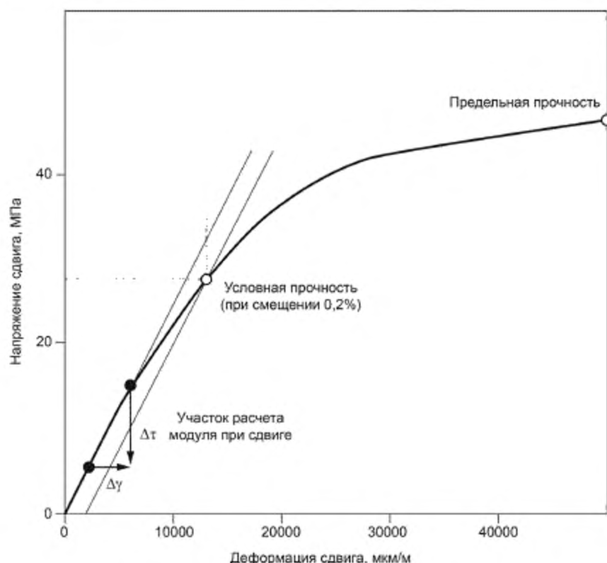
Рисунок 7 — Пример кривой «напряжение сдвига — деформация сдвига»
