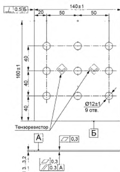
Рисунок 6 — Эскиз образца, испытываемого по методу В
