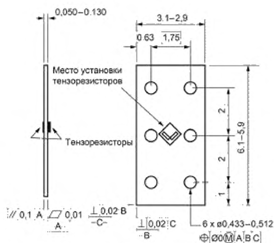
Рисунок 7 — Метод А. Образец, размеры в дюйм-фунт
