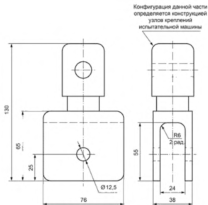
Рисунок ДА.2 — Эскиз скобы
