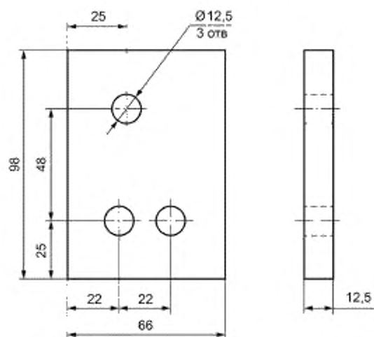
Рисунок ДА.3 — Эскиз выравнивающей пластины
