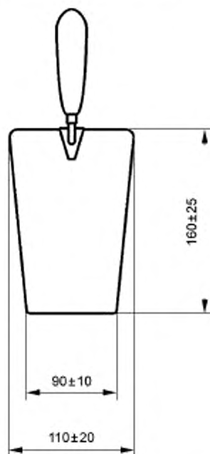
Рисунок 1 — Штукатурная лопатка
