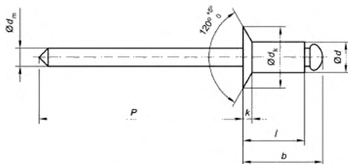
Рисунок 1 — Размеры заклепок
