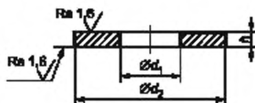
Рисунок 2 — Шайба типа L
