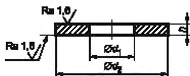
Рисунок 1 — Шайба типа N
