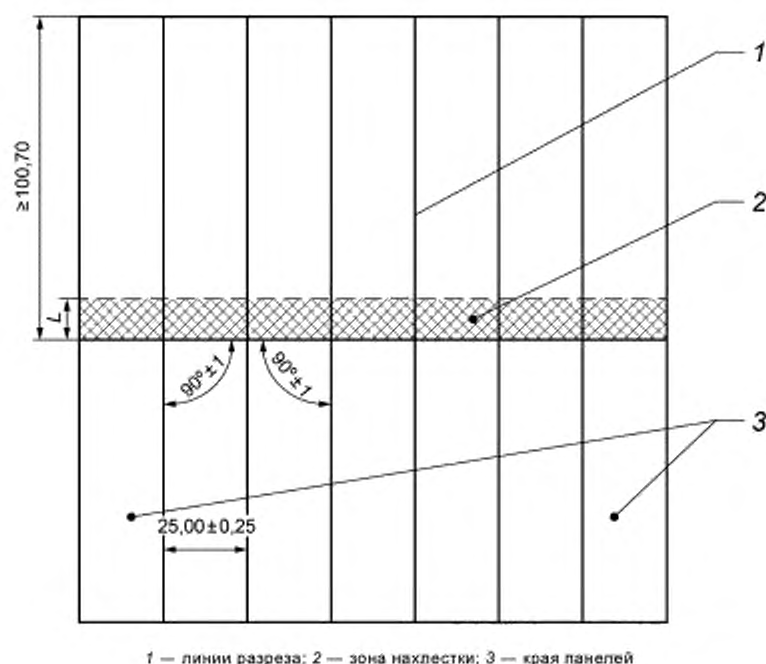
Рисунок 2 — Стандартная панель для изготовления образцов
