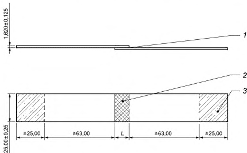
1 — клей в клеевом соединении; 2 — зона нахлестки; 3 — захватная часть образца
