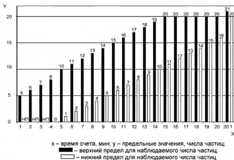
Рисунок D.2 — Графическое представление границ соответствия или несоответствия для метода последовательного отбора проб
