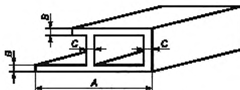
A — размер филъеры; B — толщина стенки открытого профиля; C — толщина стенки закрытого профиля
