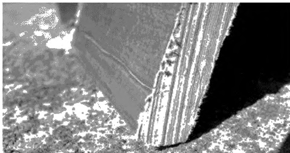
Рисунок А.7 — Волосая трещина
