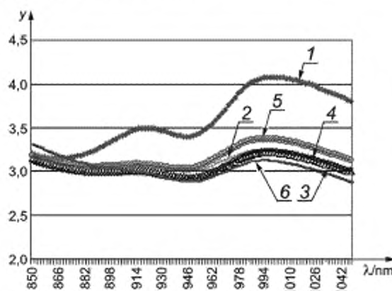
Рисунок В.2 — Спектр поглощения с x-выбросом
