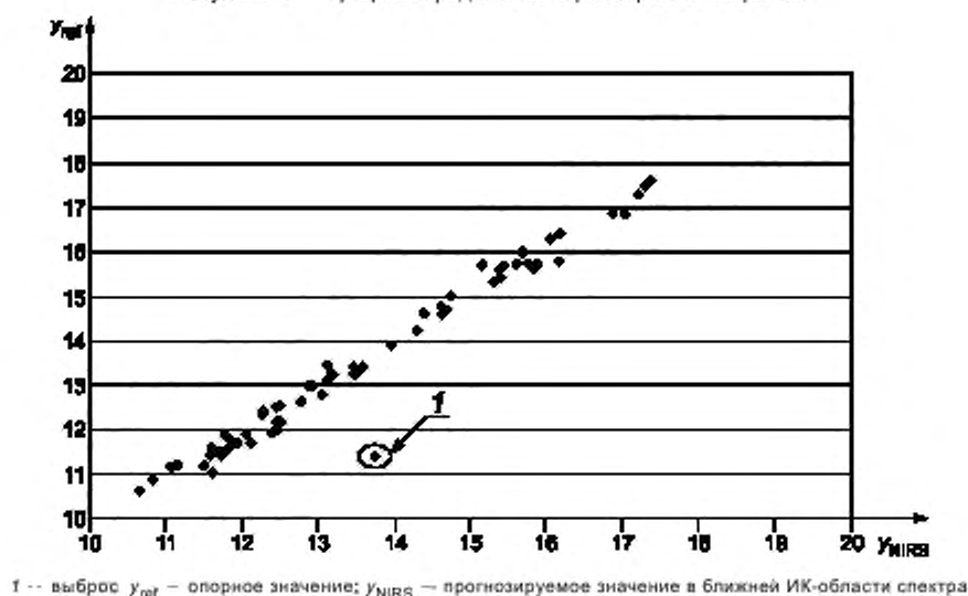
Рисунок В.4 — График рассеяния с y-выбросом
