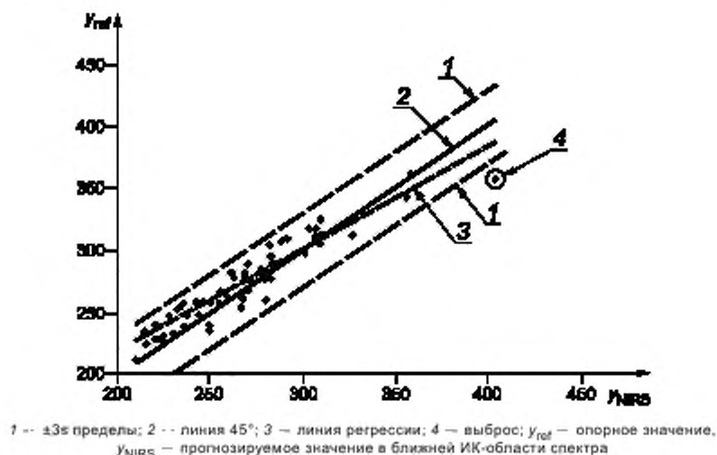
Рисунок В.5 — Пример определения ADF в зерне на кормовые цели с y-выбросом
