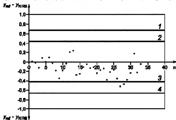
Рисунок В.5 — Пример определения ADF в зерне на кормовые цели с y-выбросом
