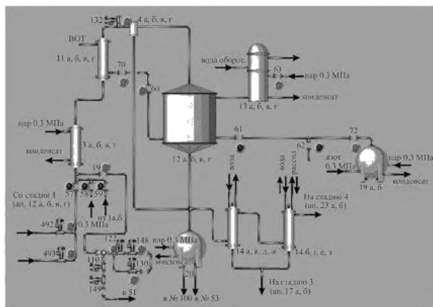
Рисунок А.2 — Виртуальный тренажер по отработке навыков по предотвращению и локализации аварийных ситуаций на химическом производстве (на примере установки синтеза монометиламина) [6]
