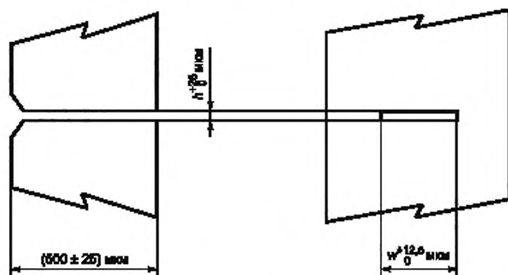
Рисунок 2 — Апертурный калибр
