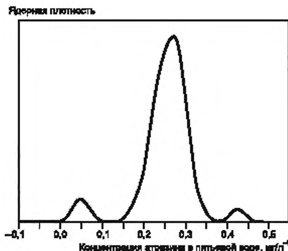
Рисунок Е.3 — График плотности по результатам участников
