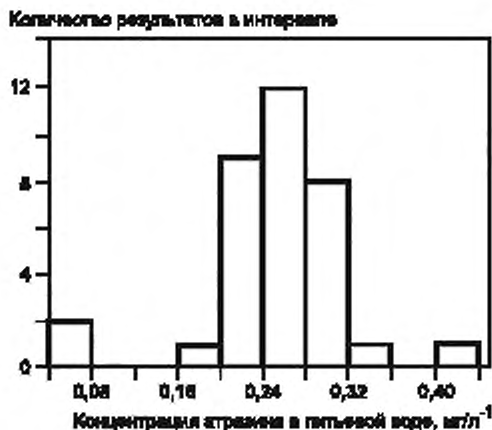
Рисунок Е.2 — Гистограмма результатов участников
