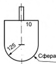
Рисунок 2 — Сбрасываемый ударник
