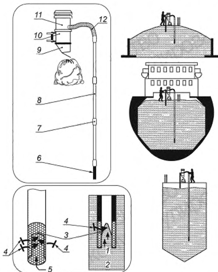
в) Пример осуществления отбора пробы на глубине более 2 м (суда, трюмы танкеров и т. д.)
