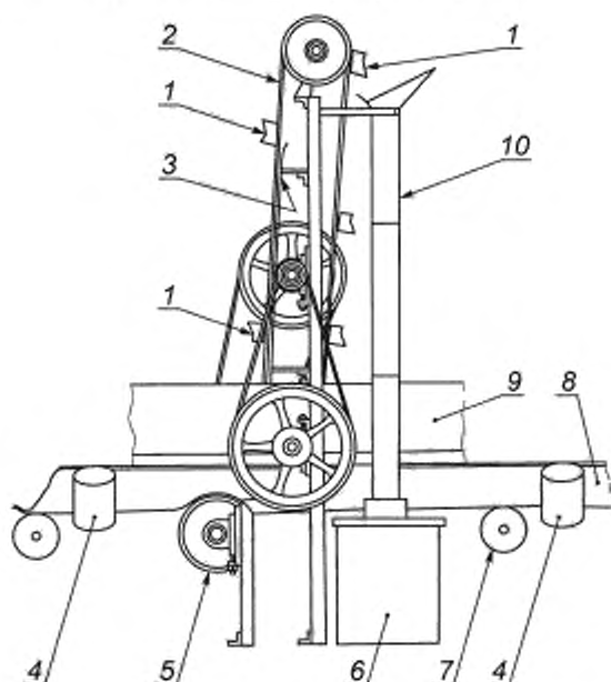
1 — ковш(и) для отбора проб; 2 — лента (цепь) с ковшом для отбора проб; 3 — направляющая цепи ковша; 4 — баланс; 5 — специальный ролик; 6 — контейнер для проб; 7 — ведущий ролик; 8 — конвейерная лента; 9 — ограждение; 10 — бункер
