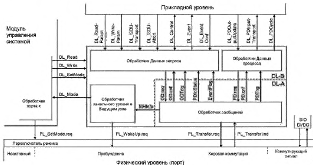
Рисунок 26 — Структура и услуги DL (Ведущий узел)
