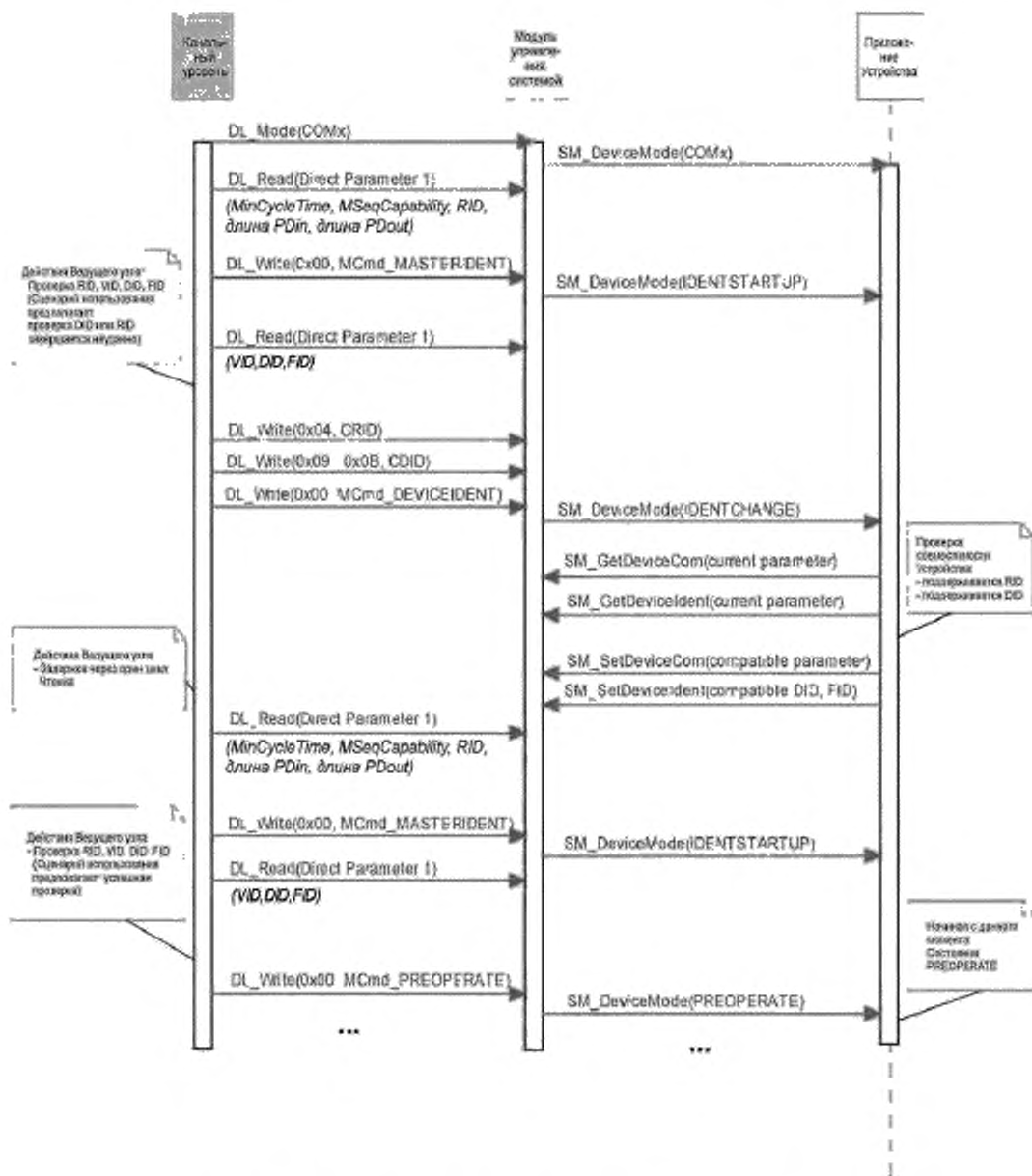
Рисунок 81 — Диаграмма последовательностей запуска Устройства в режиме совместимости
