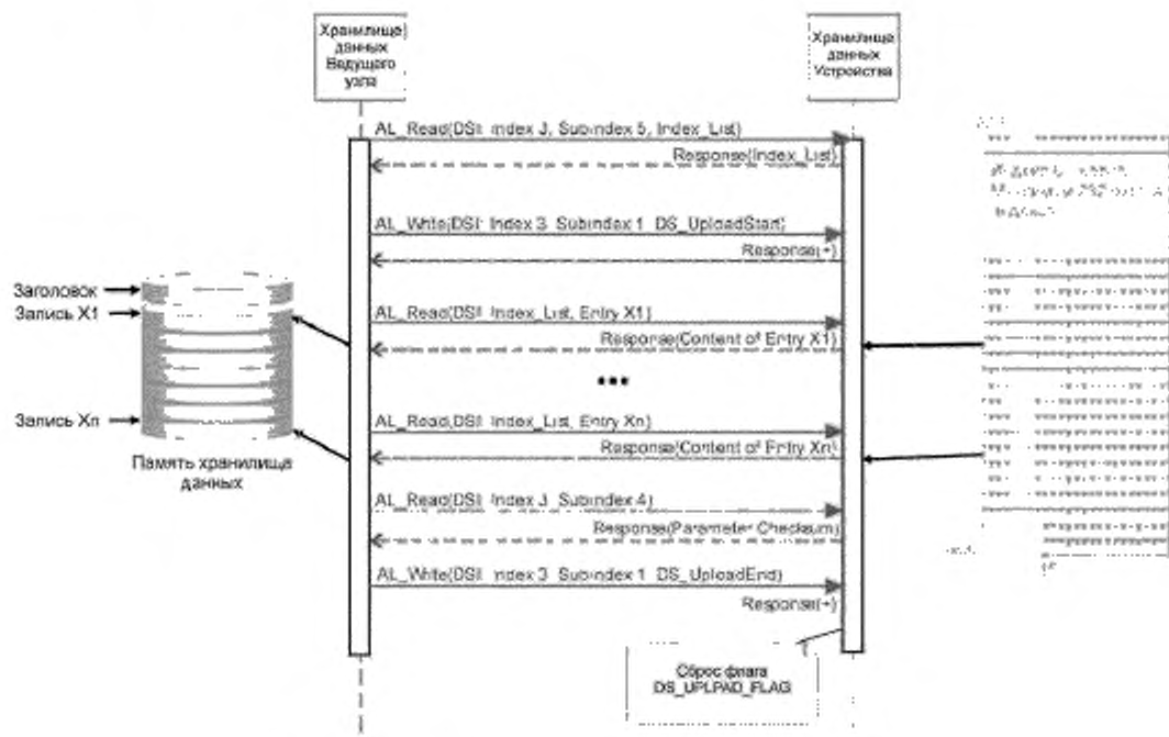
Рисунок 102 — Диаграмма последовательности подкачки в DS
