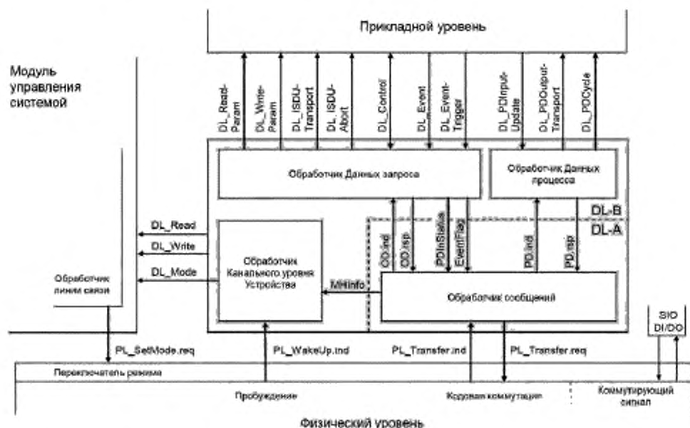
Рисунок 27 — Структура и услуги DL (Устройство)
