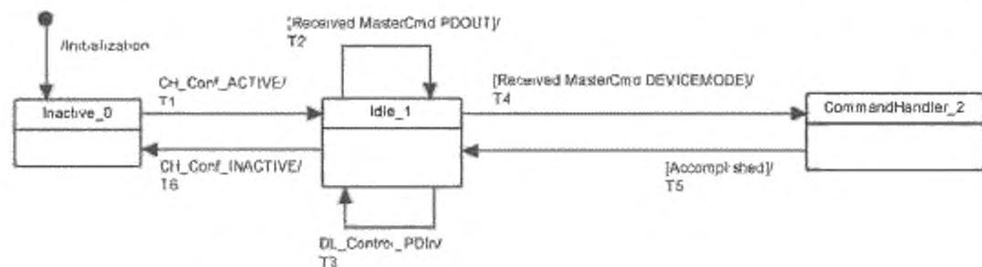
Рисунок 52 — Конечная машина обработчика команд на Устройстве
