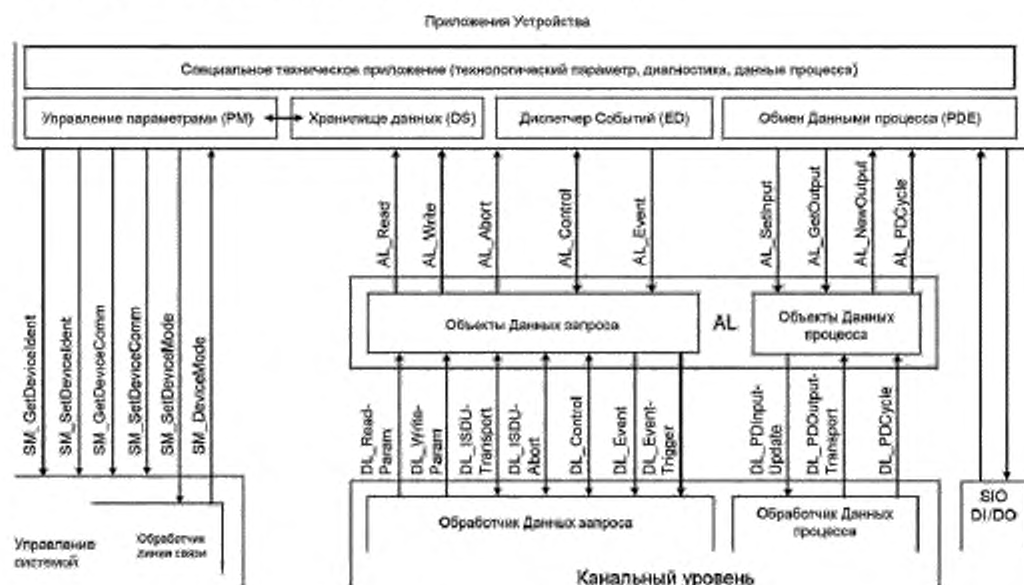
Рисунок 56 — Структура и услуги AL (Устройство)
