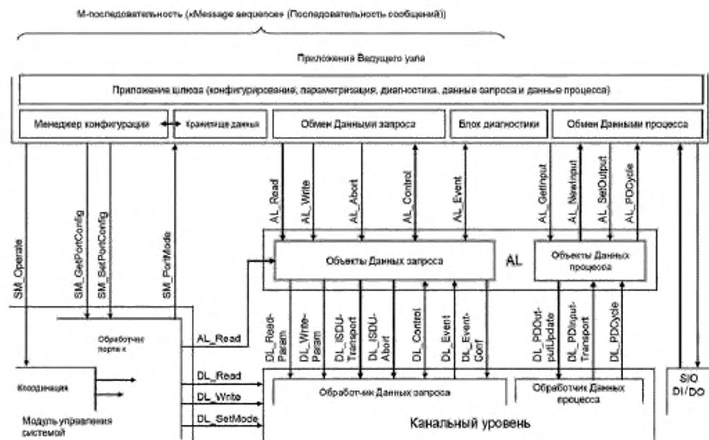
Рисунок 55 — Структура и услуги AL (Ведущий узел)
