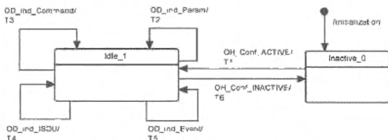
Рисунок 47 — Конечная машина обработчика OD на Устройстве
