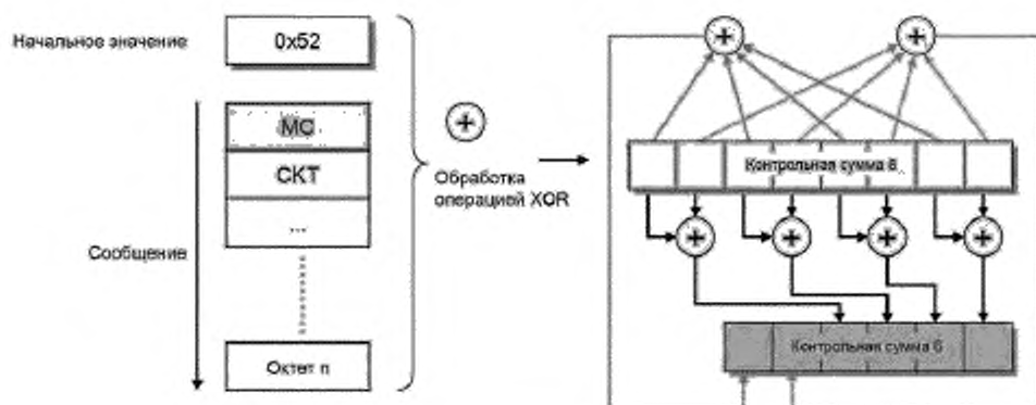
Рисунок A.4 — Принцип вычисления контрольной суммы и сжатия
