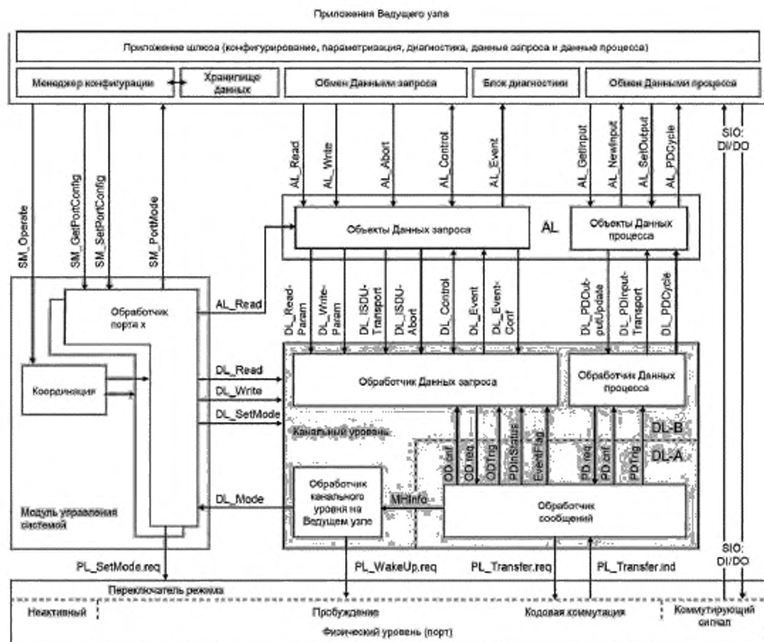
Рисунок 94 — Структура и услуги Ведущего узла
