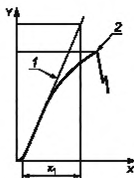
Рисунок 2 — Пример типичной кривой «нагрузка — деформация»
