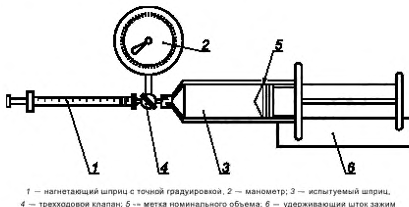
Рисунок В.1 — Испытательный стенд для определения податливости
