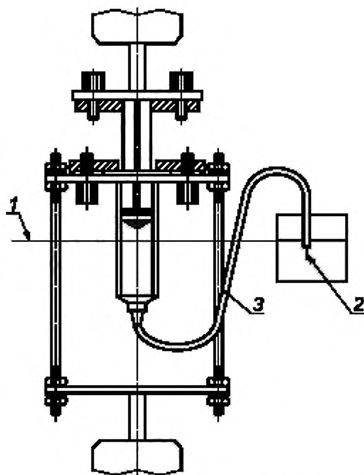
1 — уровень воды на отметке 50 % номинального объема шприца; 2 — игла (диаметром 1,2 мм (18G) и длиной приблизительно 10 см); 3 — инфузионная магистраль (полиэтиленовая трубка с внутренним диаметром 1,2 мм и длиной 1 м)
