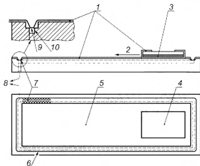
1 — испытуемая поверхность с покрытием; 2 — тензодатчик; 3 — пористая резина; 4 — салазки; 5 — горизонтальная платформа; 6 — вакуумный зажим; 7 — проволочная сетка с мелкими отверстиями; 8 — вакуумный насос; 9 — проволочная сетка; 10 — канал с разреженным воздухом
