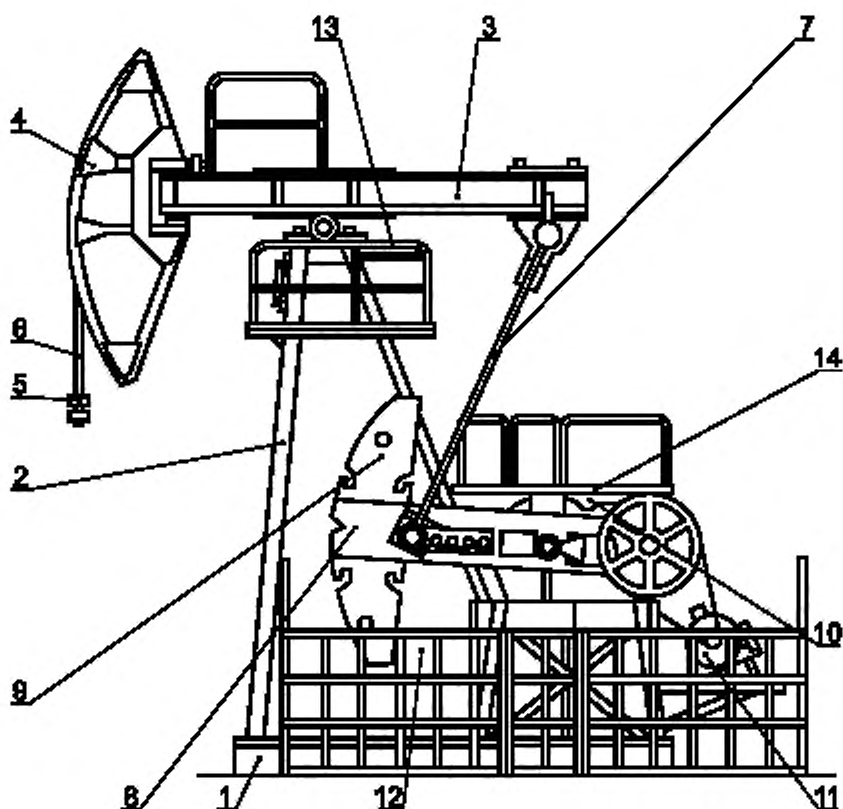
1 — рама; 2 — стойка; 3 — балансирующий рычаг; 4 — головка балансирующего рычага; 5 — подвеска устьевых штоков; 6 — траверса; 7 — шатун; 8 — кривошип; 9 — уравновешивающее устройство с использованием грузов или пневматического аккумулятора; 10 — редуктор; 11 — приводной двигатель (электрический двигатель или двигатель внутреннего сгорания); 12 — защитное ограждение; 13 — верхняя площадка; 14 — смотровая площадка
