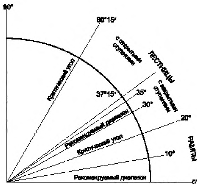
Рисунок 1 — Углы наклона средств доступа к рабочему месту
