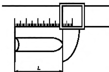
Рисунок 2 — Измерения штангенциркулем длины пеллеты между средней точкой выпуклого конца пеллеты и вогнутым поперечным сечением пеллеты
