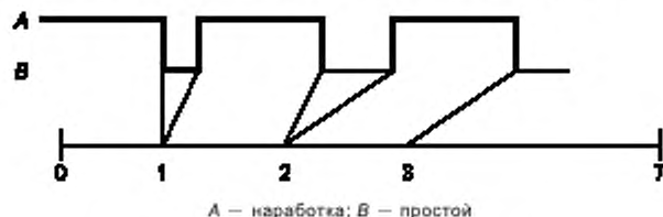
Рисунок 1 — Один восстанавливаемый объект
