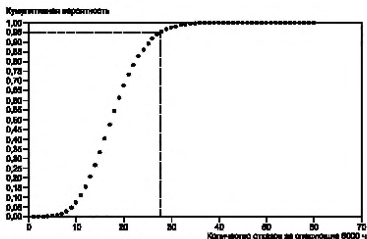
Рисунок С.5 — График кумулятивной функции апостериорного распределения вероятностей количества отказов M
