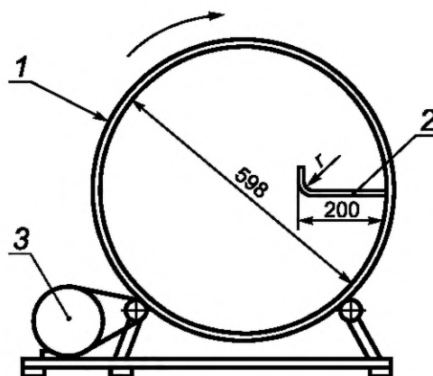
1 — барабан; 2 — перегородка; 3 — мотор
