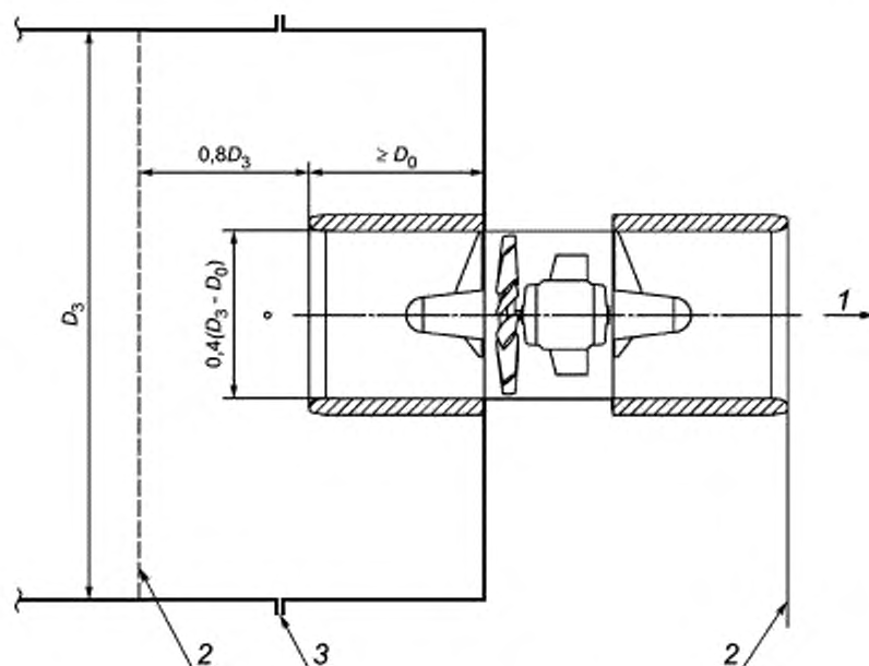
1 — направление потока, 2 — экран, 3 — приемники давления для измерения давления p_{вз}
