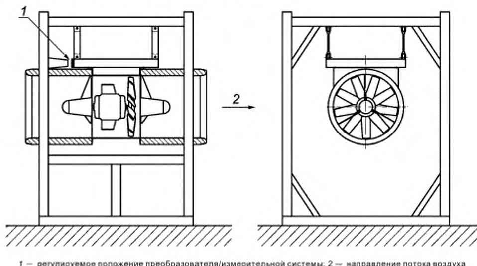
Рисунок 2 — Схема подвесного стенов, пример 1
