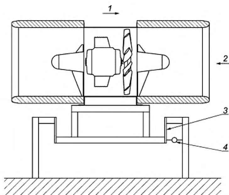
1 — направление перемещения вентилятора, 2 — направление потока воздуха; 3 — листовая рессора; 4 — датчик силы
