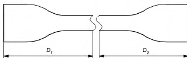
Рисунок А.2 — Измерение положения места разрушения
