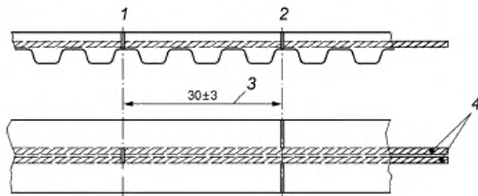
1 — разрезают два корда, 2 — разрезают все, кроме двух кордов; 3 — расстояние между разрезами; 4 — корды
