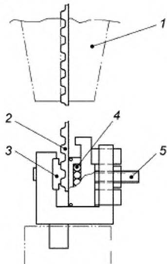
1 — зажим разрывной машины; 2 — образец; 3 — приспособление для сдвига зуба; 4 — подшипник скольжения; 5 — установочный болт
