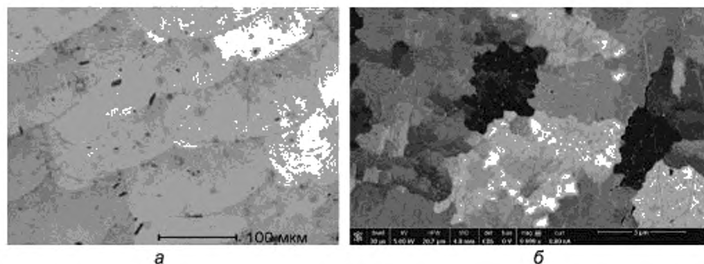
Рисунок 3 — Фронты кристаллизации (а) и ячейки (б) структуры образца
