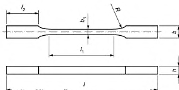
l — длина образца; l_1 — длина рабочей части образца; l_2 — длина захватов; b — ширина образца; b_1 — ширина рабочей части образца; h — толщина образца; R — радиус закругления
