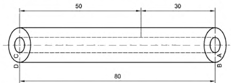
Рисунок В.1 — Форма и размеры образца
