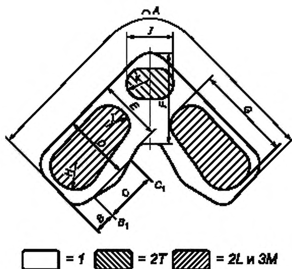
Рисунок 4 — Вид сверху на внешнюю поверхность бахилы, на котором изображены размеры защитных зон в соответствии с таблицами 5 и 6. Для отчетливости язычок не изображается.
