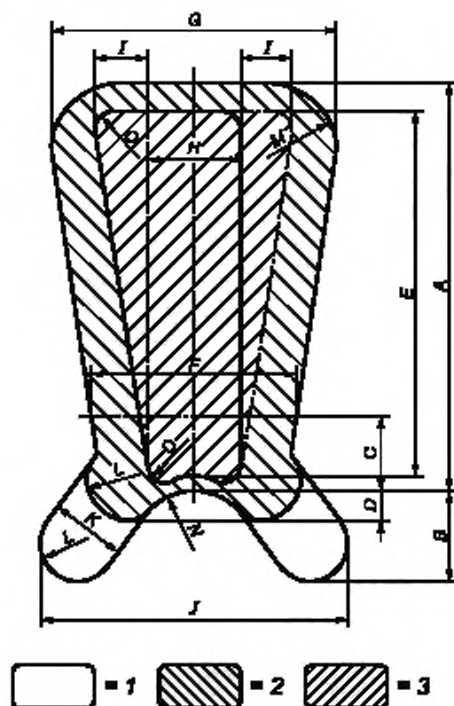
1 — зона 1, область лодыжек; 2 — зона 2, внешняя область; 3 — зона 3, внутренняя область
