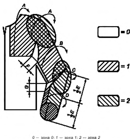
Рисунок 9 — Схема одежды, содержащей наплечники, налокотники и нарукавники, на которой показаны названные размеры (см. таблицу 11)
