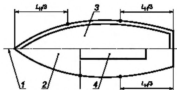
1 — диаметральный плоскость; 2 — палуба; 3 — открытое судно; 4 — кокпит
