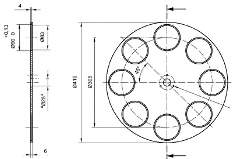
б) Вид сверху и сечение
