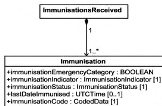
Рисунок 5 — Структура класса ImmunisationsReceived
