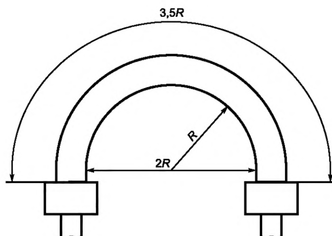
Рисунок 3 — Схема изгиба рукавов при динамических испытаниях
