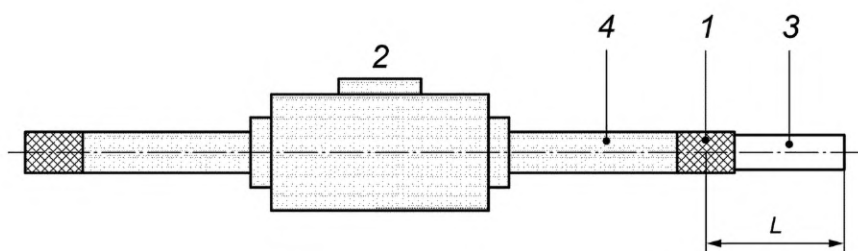
с) Образец (например, клапан) в сборке с патрубком
