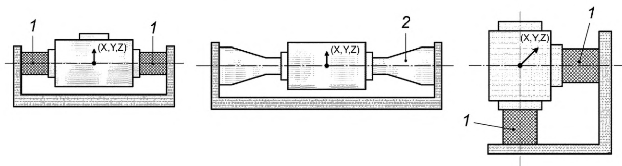
Рисунок 7 — Монтаж компонентов на вибростенде
