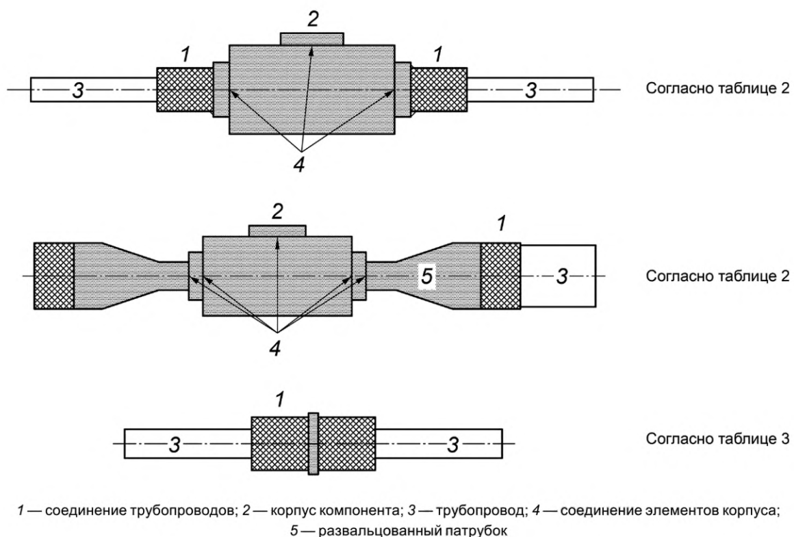
Рисунок 1 — Виды соединений компонентов и трубопроводов
