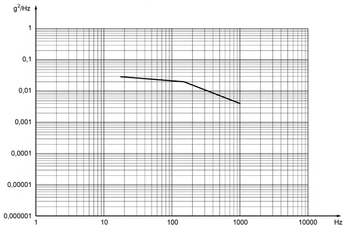
Рисунок 8 — Спектральная плотность мощности
