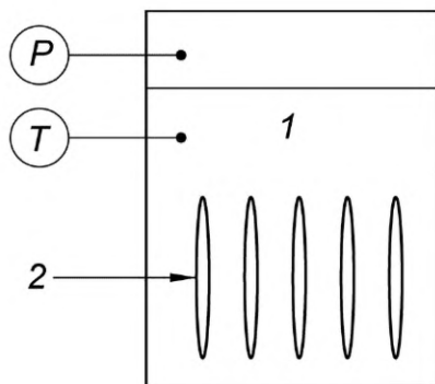
1 — жидкий хладагент; 2 — испытываемые образцы; P — давление; T — температура
