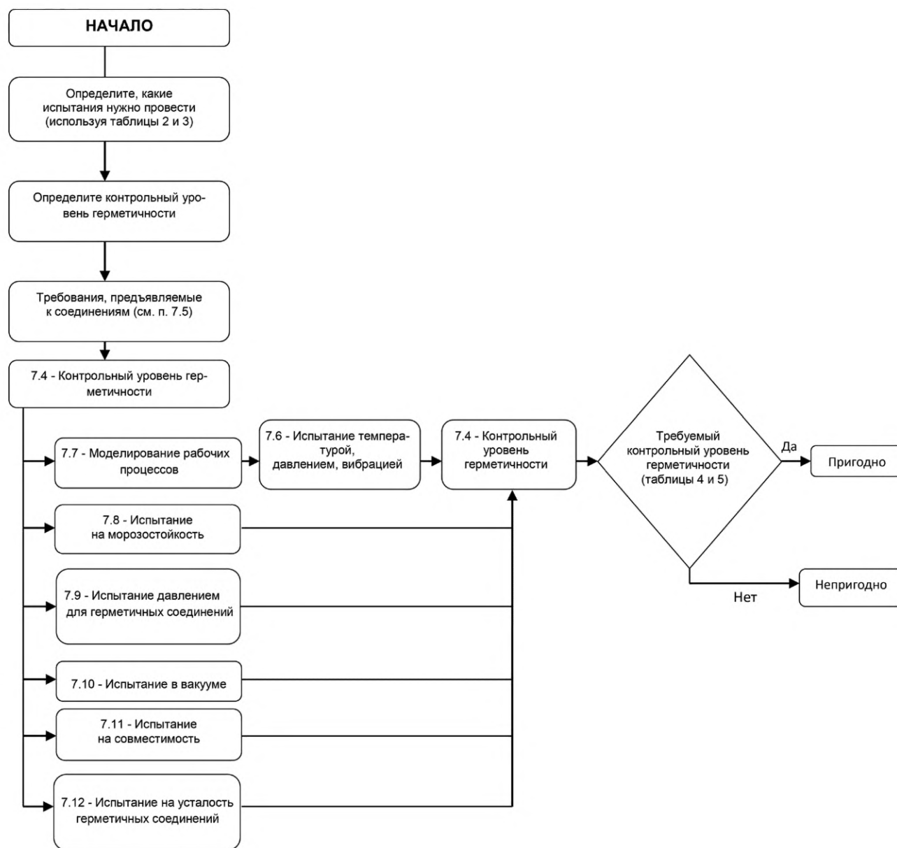
Рисунок 2 — Последовательность испытаний
