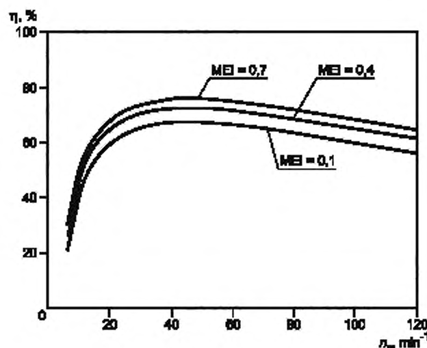
Рисунок 4 — Зависимости КПД от n_v , полученные для консольного насоса (тип К) с частотой вращения вала n_N = 2900 \text{ мин}^{-1} , подачей Q_{BEP} = 32 \text{ м}^3/\text{ч} и различными значениями MEI
