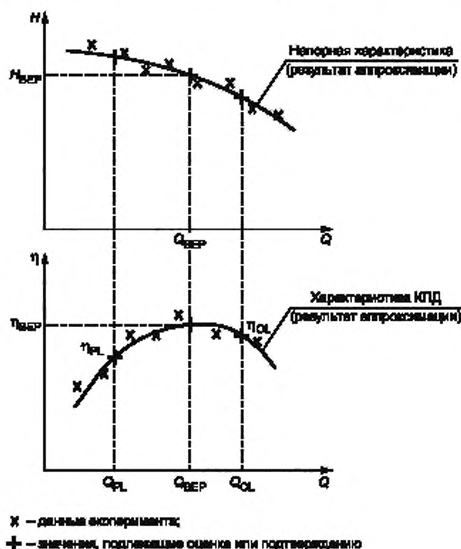
Рисунок 5 — Совмещенное графическое представление экспериментальных данных и аппроксимирующих функций
