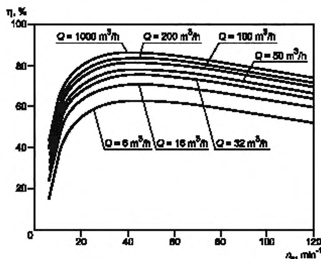
Рисунок 3 — Зависимости КПД от n_v , полученные для консольного насоса (тип К) с частотой вращения вала n_N = 2900 \text{ мин}^{-1} , MEI = 0,7 и различными значениями Q_{BEP}
