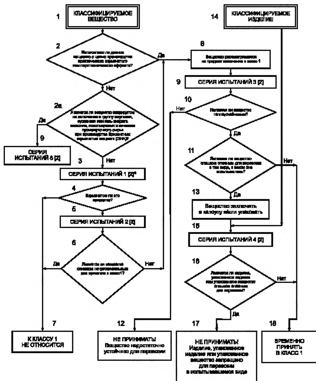
Рисунок Б.8 — Схема процедуры временного принятия вещества или изделия в класс 1.
