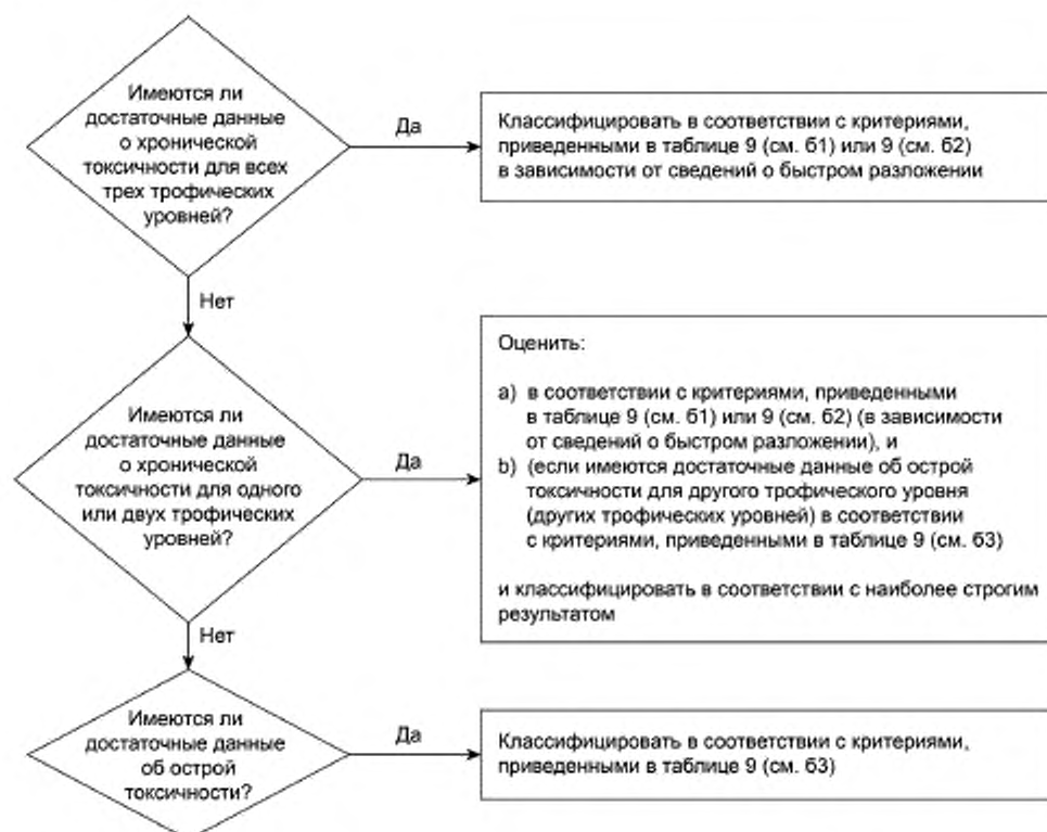
Рисунок Б.4 — Категории веществ, характеризующихся длительно действующей опасностью для водной среды
