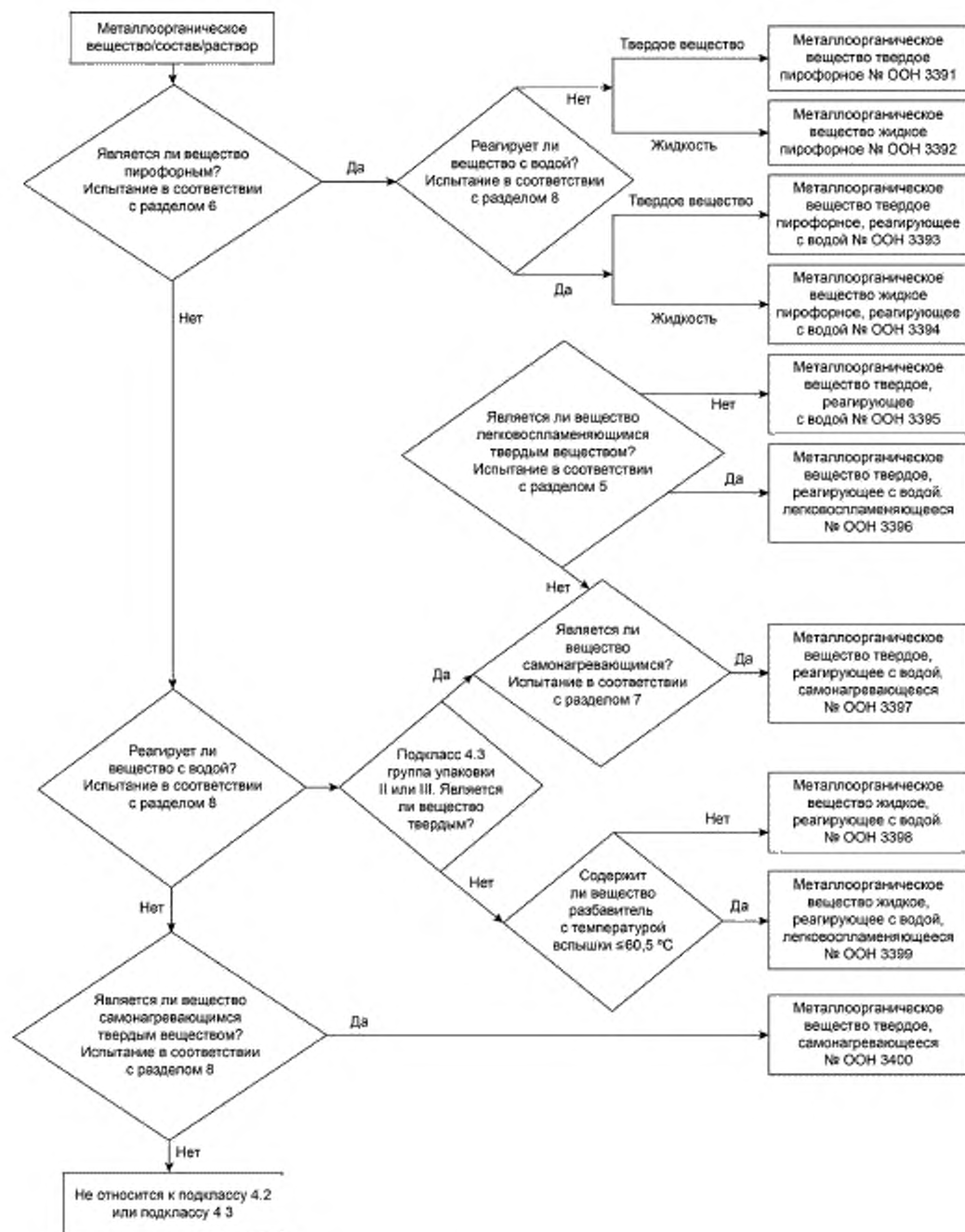
Рисунок Б.3 — Схема классификации металлоорганических веществ
