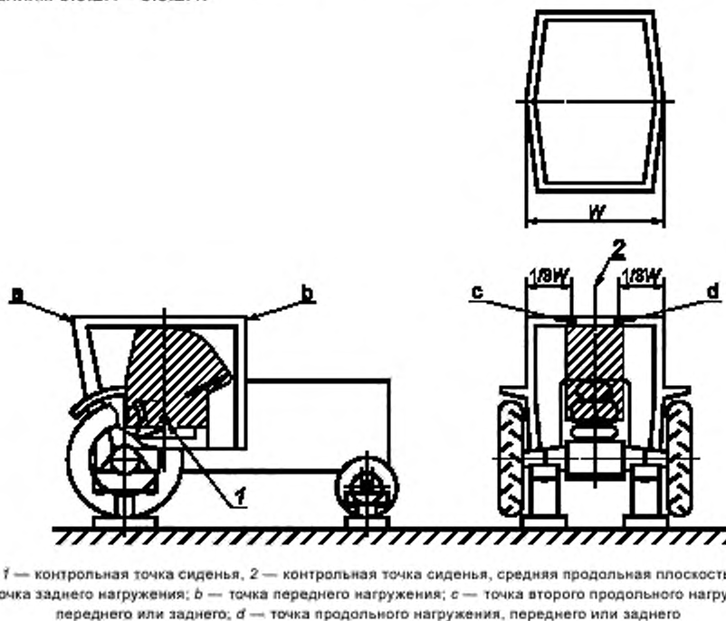
Рисунок 8 — Переднее и заднее нагружение
