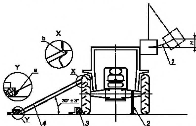
1 — траектория перемещения центра тяжести маятникового блока, проходящая через точку удара; 2 — крепления трактора (5.2.3); 3 — брус из мягкой древесины сечением 150 × 150 мм; 4 — деревянный упор; a — заостренный торец упора; b — скругленный торец упора для обеспечения контакта с ободом колеса
