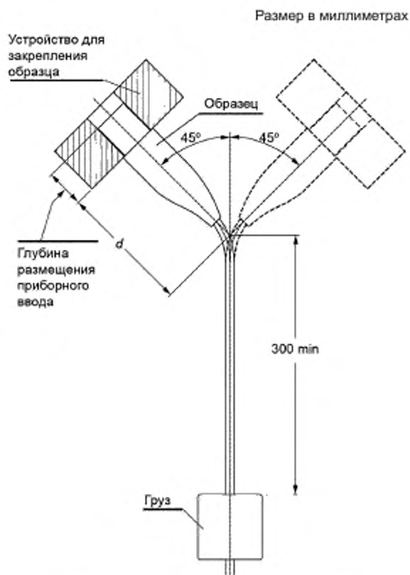
Рисунок 2 — Устройство для испытания на изгиб
