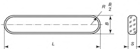
Рисунок 1 — Стекло рифленое
