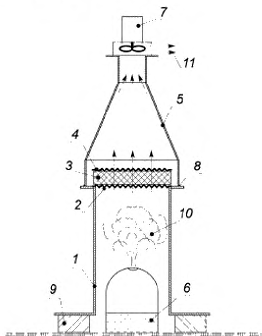
1 — воздухопроницаемая основа; 2 — нижняя опорная сетка; 3 — образец для испытаний; 4 — верхняя прижимная сетка; 5 — воздухопроницаемый колпак; 6 — электропароувлажнитель; 7 — воздушный насос; 8 — резиновые уплотнители; 9 — подставки под основание; 10 — паровоздушная смесь; 11 — отработанная паровоздушная смесь
