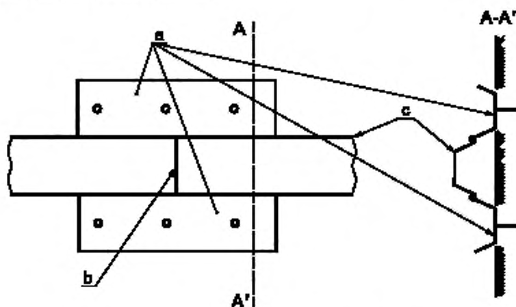
a — протяжный шаблон, закрепленный на опоре; b — стыковое соединение; c — части длинного элемента, подлежащие сварке
