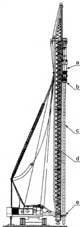
а — молот, б — оголовок шпунта; с — шпунтовая свая, d — направляющая стрела копра; е — нижняя направляющая
