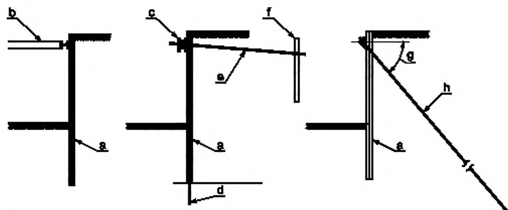
а — шпунтовая свая; б — жесткий элемент; с — пояс; d — скальный дюбель; e — стержень анкера; f — анкерная плита или анкерная стенка; g — переменный угол; h — запрессовываемый анкер или свая, работающая на растяжение
