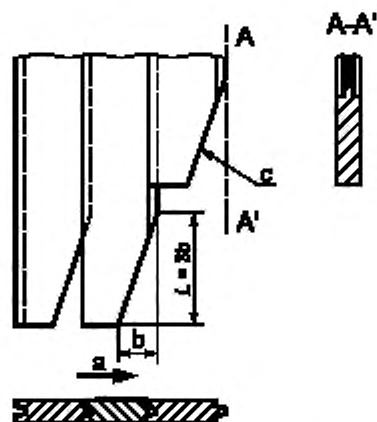
a — направление установки, b — ширина снятой фанки, c — направление давления грунта
