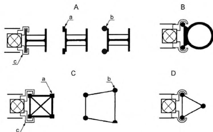
А — несущая направляющая стрела копра; В — трубчатая направляющая стрела копра; С — направляющая стрела копра в виде решетчатой опоры; D — треугольная направляющая стрела копра; а — четырехугольный полый профиль, b — труба; с — направляющая стрела копра
