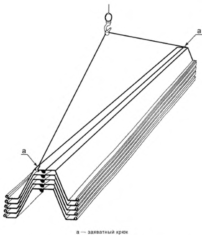
Рисунок А.2 — Подъем шпунтовых свай без траверсы
