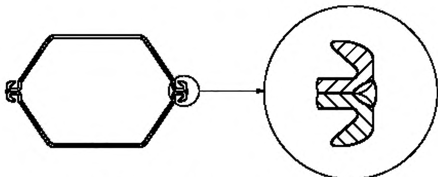
Рисунок 7k — Продольный шов сборных свай коробчатого сечения
