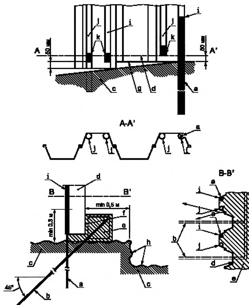
а — скальный дюбель, б — наклонный скальный анкер в случае выемки скальной породы перед шпунтовой стенкой; с — естественная скальная порода, d — шпунтовая свая, e — железобетонная балка; f — очищенная поверхность; g — глубина подошвы шпунтовой сваи; h — вырытый котлован в скальной породе; i — труба прикреплена в том месте, где ожидается наименьшее расстояние между шпунтовой свайей и скальной породой; j — резервная труба; k — пробка из бетона, которую следует создать перед установкой
