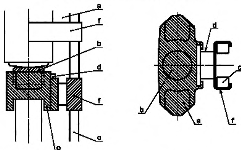
а — молот, б — амортизирующая прокладка оголовка шпунта, с — направляющая стрела копра, д — направляющая скольжения, е — оголовок шпунта, ф — направляющая стрелы копра
